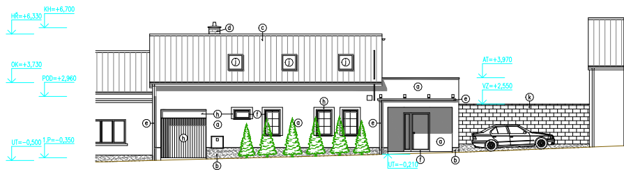
POHLED SEVERNÍ
