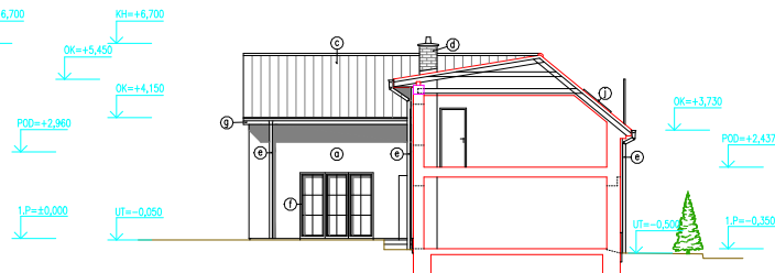
POHLED VÝCHODNÍ
