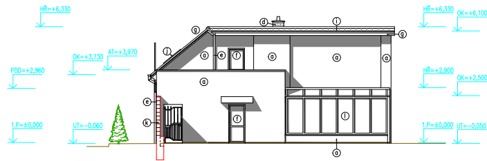
POHLED ZÁPADNÍ
